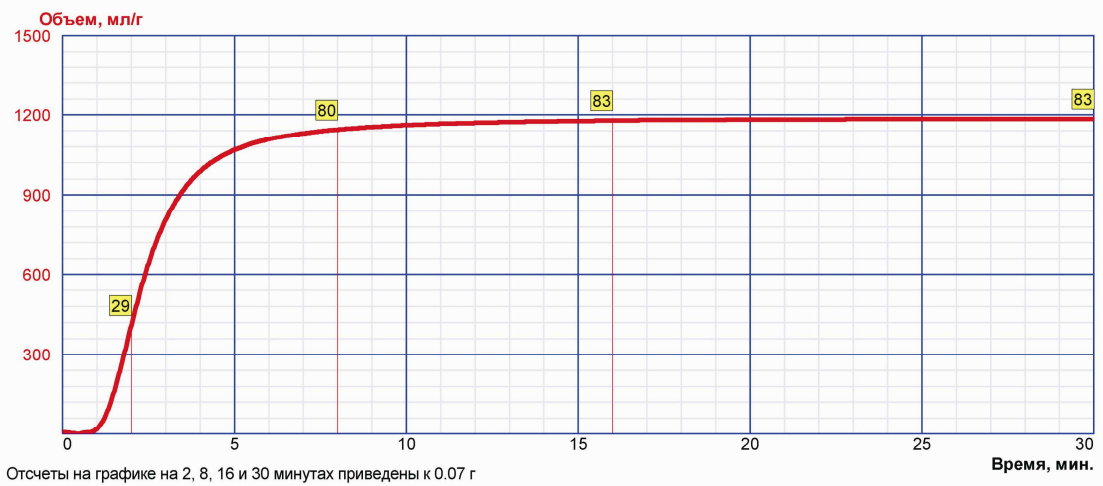
Рисунок 3 Кинетика выделения водорода ГазобетоПЛЮС
