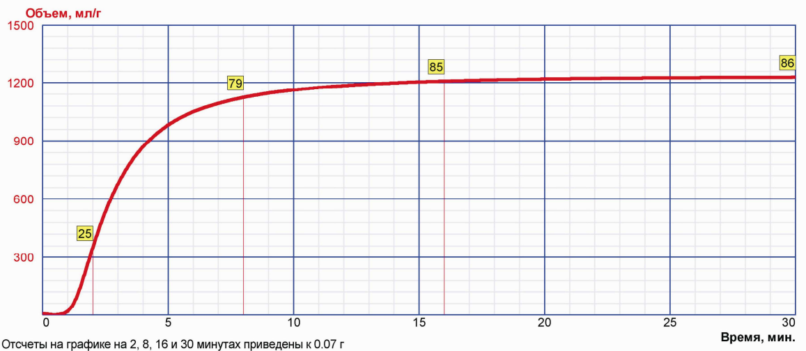
Рисунок 2 Кинетика выделения водорода Газобетопласт
